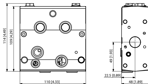
PVB 32 dimensions
